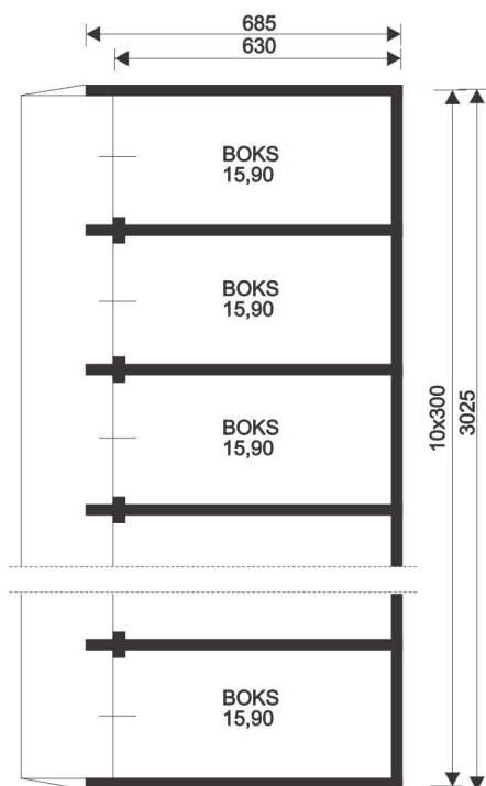
RZUT PRZYZIEMIA
