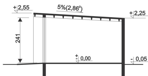
PRZEKRÓJ
