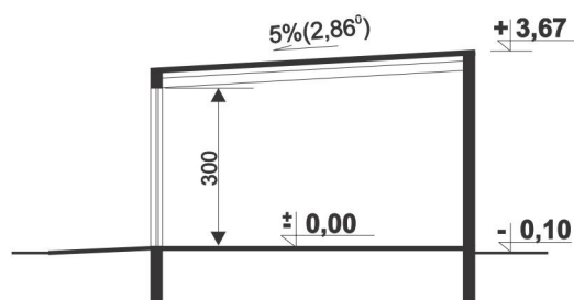
PRZEKRÓJ
