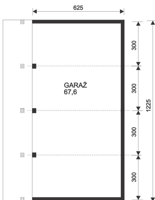
RZUT PRZYZIEMIA
