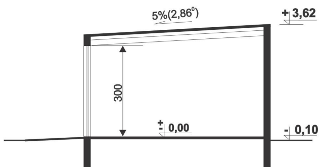
PRZEKRÓJ
