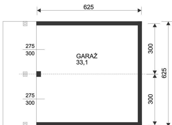
RZUT PRZYZIEMIA
