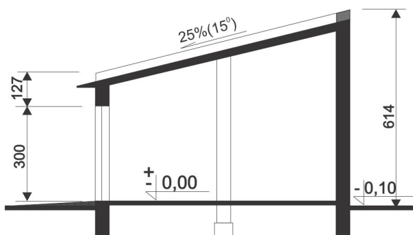
PRZEKRÓJ
