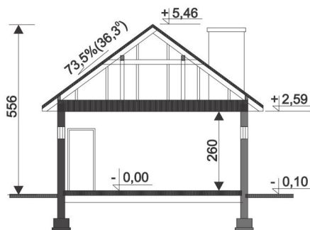
PRZEKRÓJ
