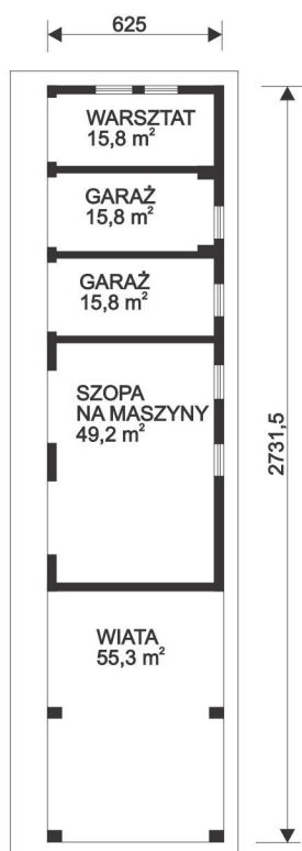
RZUT PRZYZIEMIA
