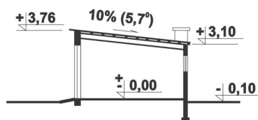
PRZEKRÓJ
