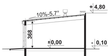
PRZEKRÓJ
