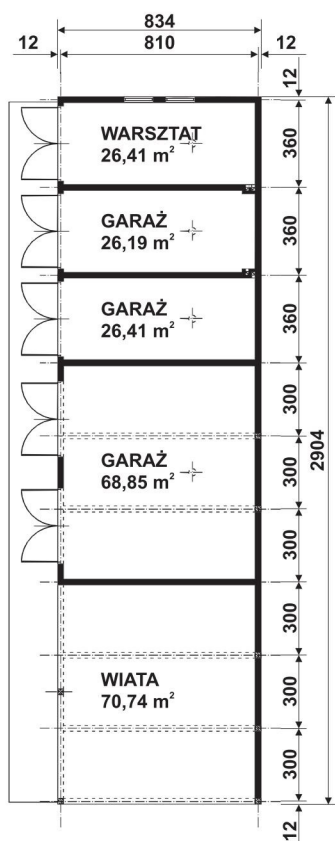
RZUT PRZYZIEMIA
