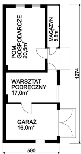
PRZYZIEMIE
