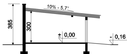
PRZEKRÓJ
