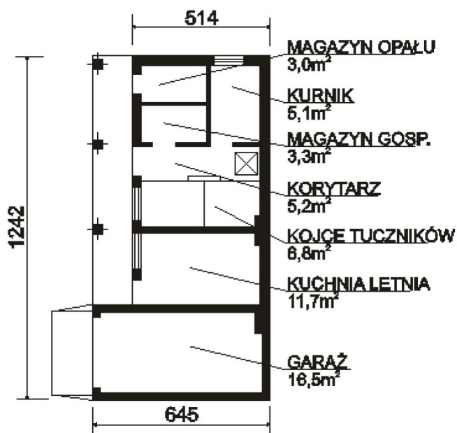
PRZYZIEMIE
