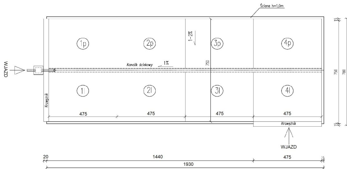
RZUT
