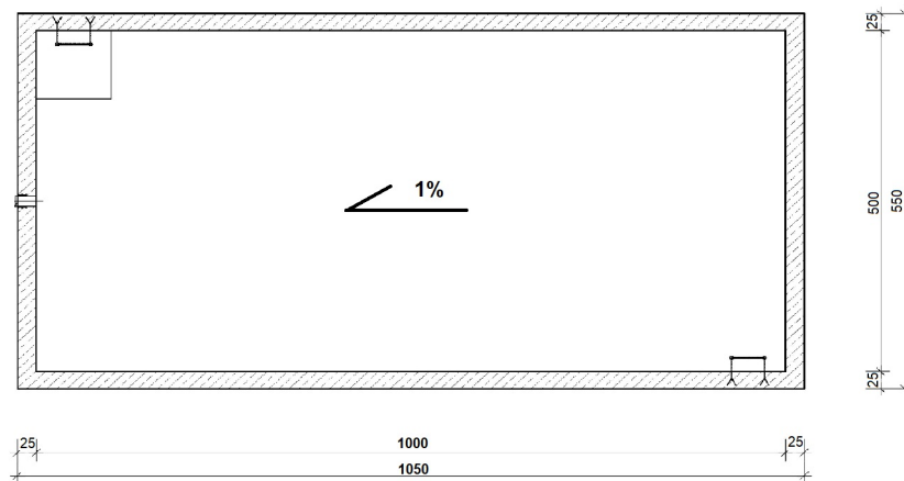
RZUT
