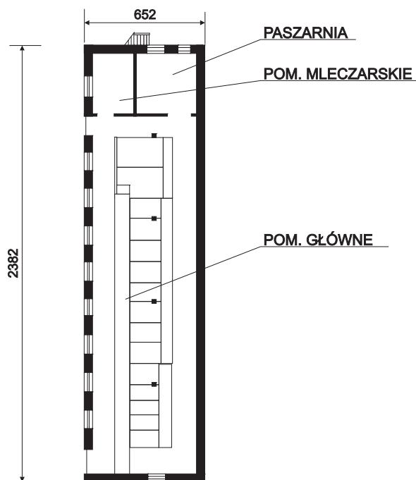
RZUT PRZYZIEMIA
