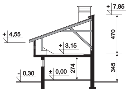
PRZEKRÓJ
