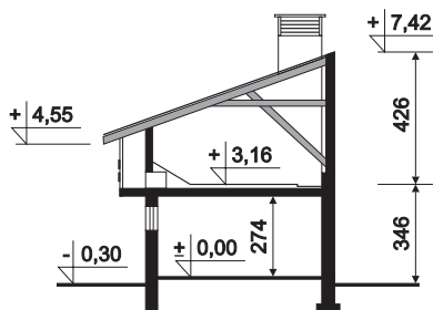
PRZEKRÓJ
