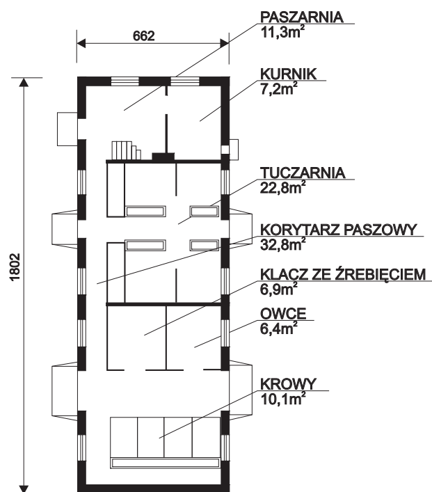
RZUT PRZYZIEMIA
