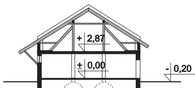
PRZEKRÓJ
