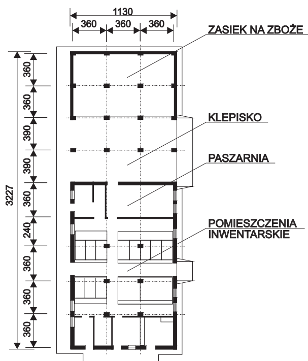
RZUT PRZYZIEMIA
